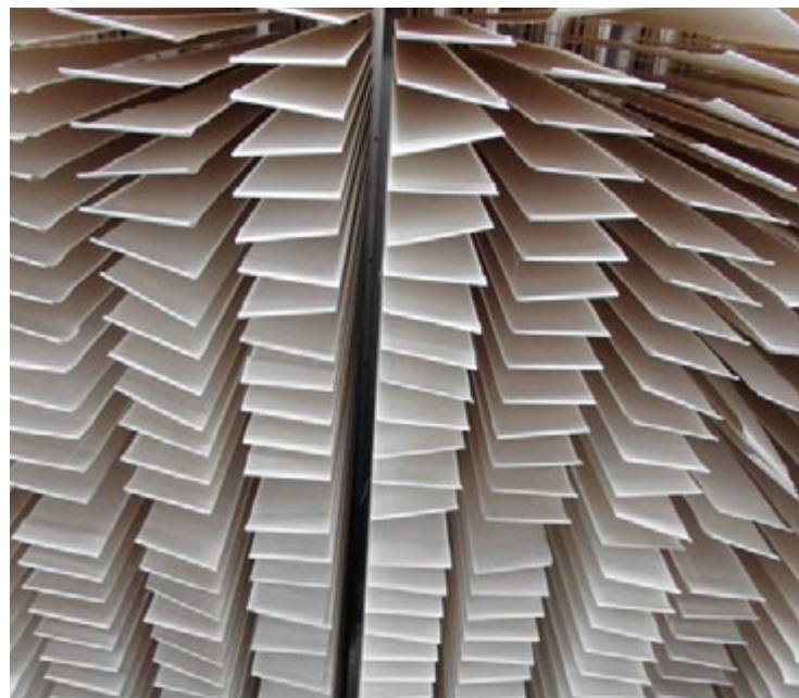
Im Lamellen-Trockenraum ist Platz für 5 000 Stück. Eine Luftumwälzung sorgt für gleichmäßige Austrocknung
